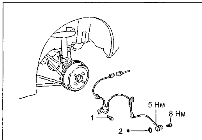
Снятие датчиков частоты вращения задних колес. 1 - датчик частоты вращения заднего левого колеса, 2 - кольцевое уплотнение.
