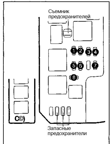
Расположение предохранителей блока в подкапотном пространстве автомобиля.
