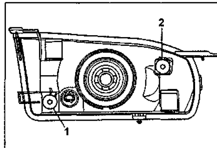
1 - вертикальная регулировка, 2 - горизонтальная регулировка.
