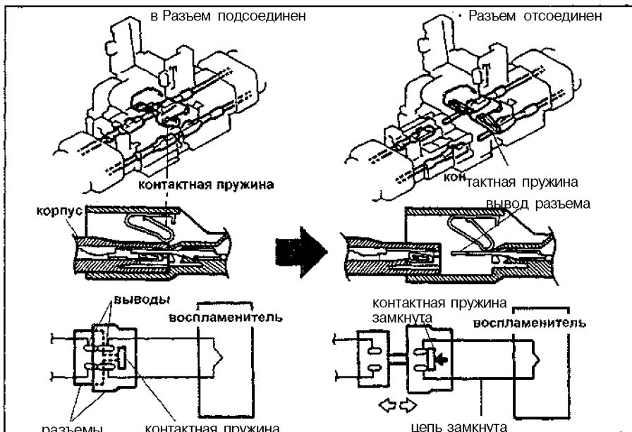
Механизм предотвращения срабатывания системы SRS.
