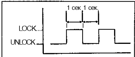
Режим перезаписи.
