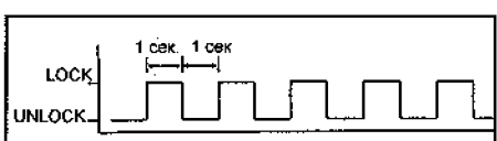
Режима стирания.
