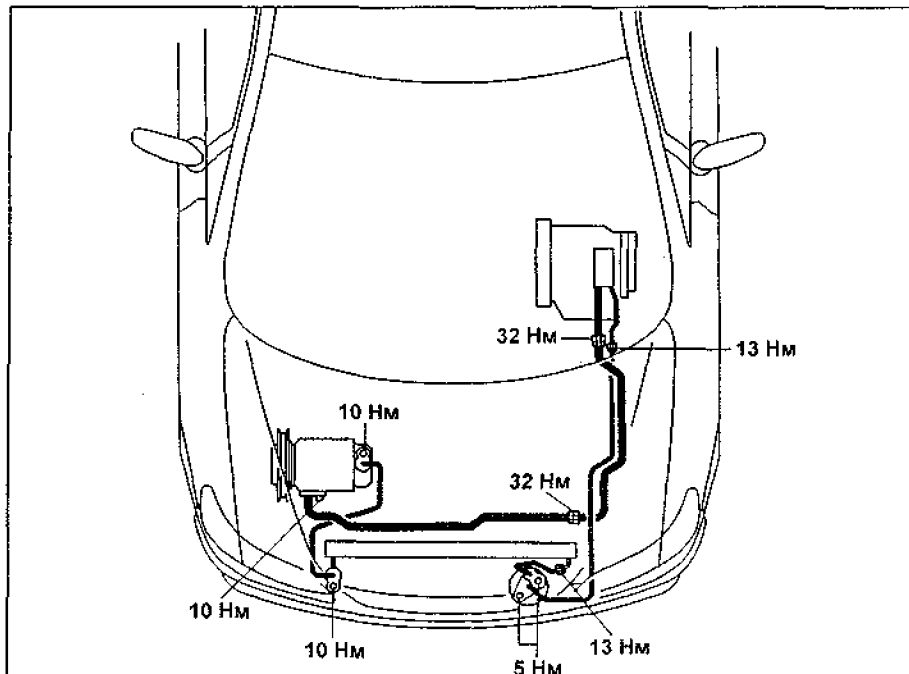
Моменты затяжки резьбовых соединений системы кондиционирования и отопления.
