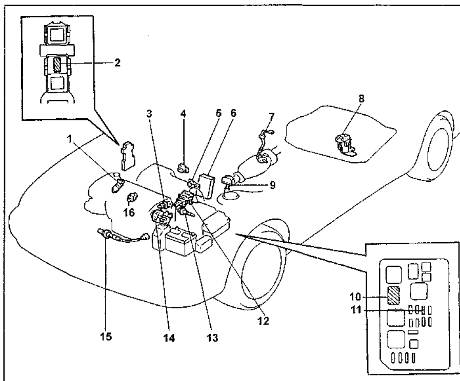
Расположение компонентов системы электронного управления. 1 - форсунка, 2 - реле-выключатель топливного насоса, 3 - датчик температуры охлаждающей жидкости, 4 - датчик абсолютного давления во впускном коллекторе, 5 - датчик положения дроссельной заслонки, 6 - электронный блок управления, 7 - датчик температуры отработавших газов (4A-FE), 8 - топливный насос, 9 - диагностический разъем, 10 - главное реле системы впрыска, 11 - предохранитель "EF!" (15A), 12 - клапан системы управления частотой вращения холостого хода, 13 - датчик температуры воздуха на впуске, 14 - объединенный узел зажигания, 15 - кислородный датчик.
