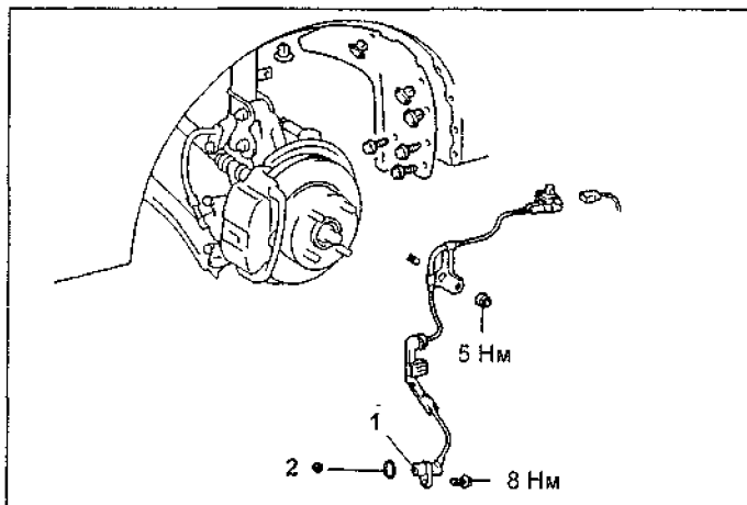
Снятие датчиков частоты вращения передних колес. 1 - датчик частоты вращения переднего левого колеса, 2 - кольцевое уплотнение.
