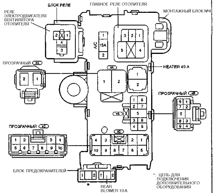
МОНТАЖНЫЙ БЛОК №4 (ВНУТРЕННИЕ ЦЕПИ)
