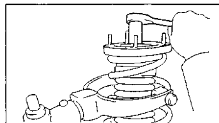
в) Отверните гайку.
