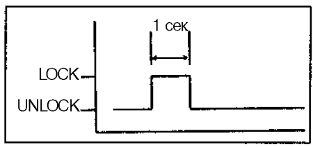
Режим добавления.
