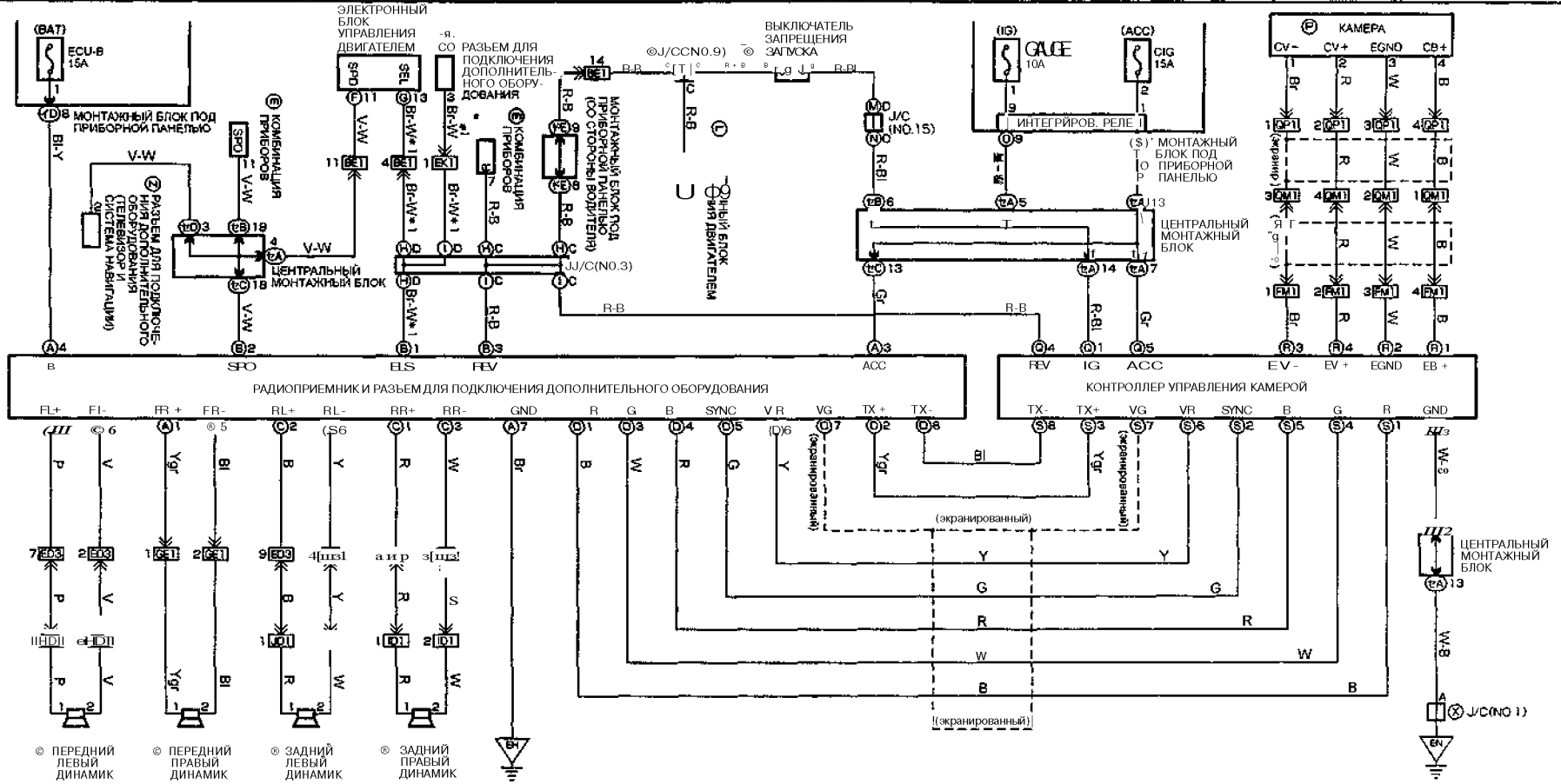
Схемы электрооборудования
