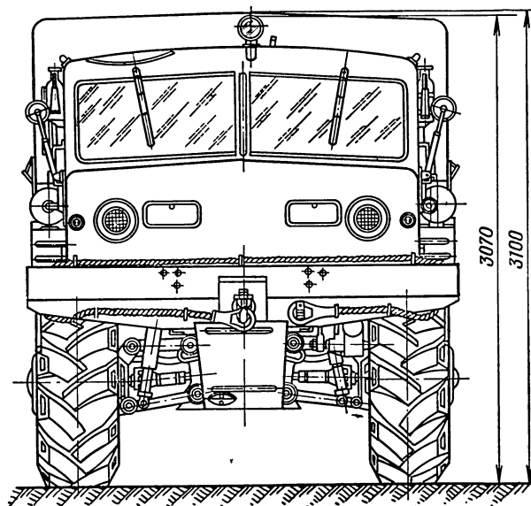
Автомобиль-тягач МАЗ-535А
