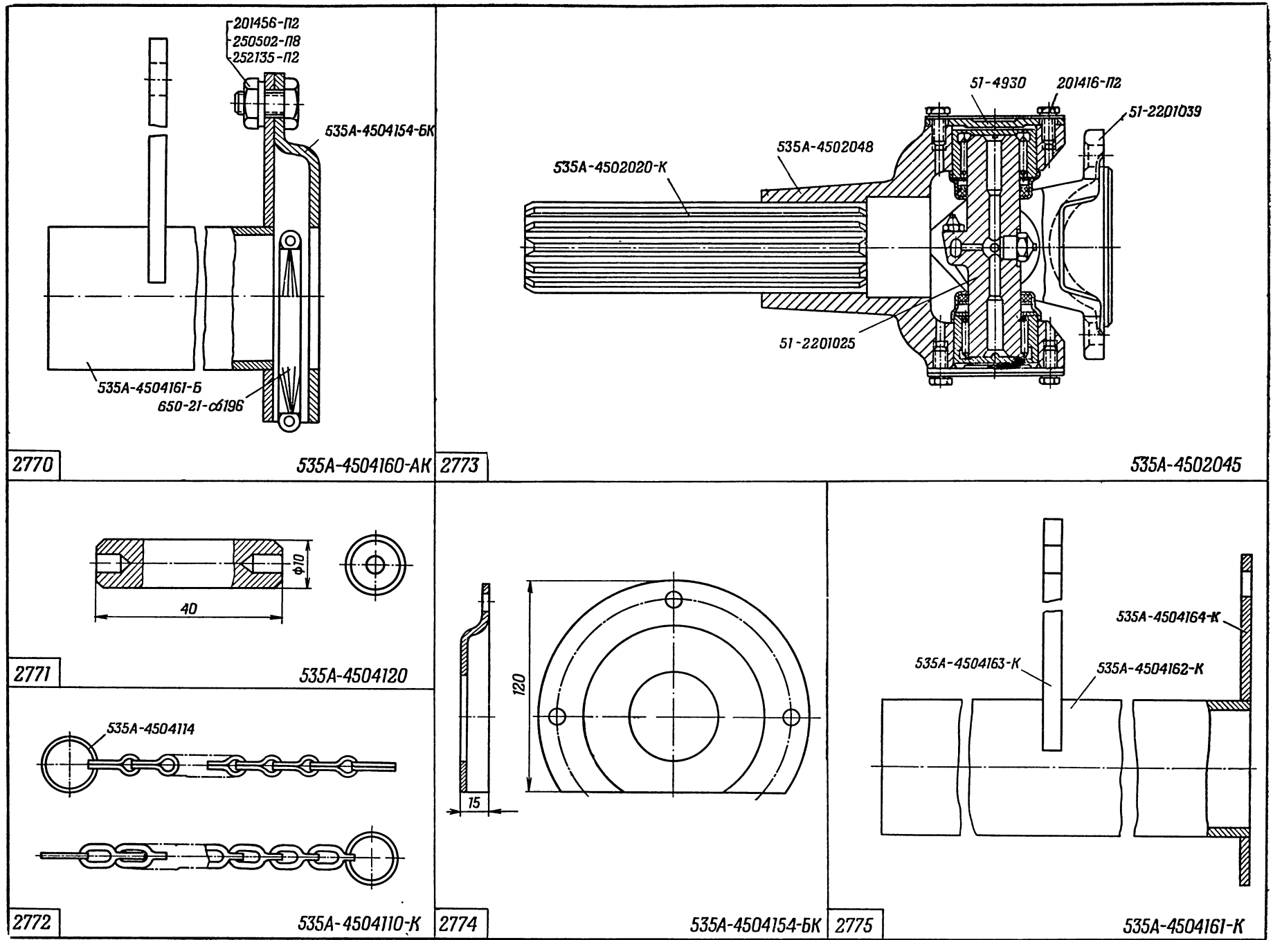
На рис. 2770 вместо дет. 535A-4504161-Б читать дет. 535A-4504161-К
