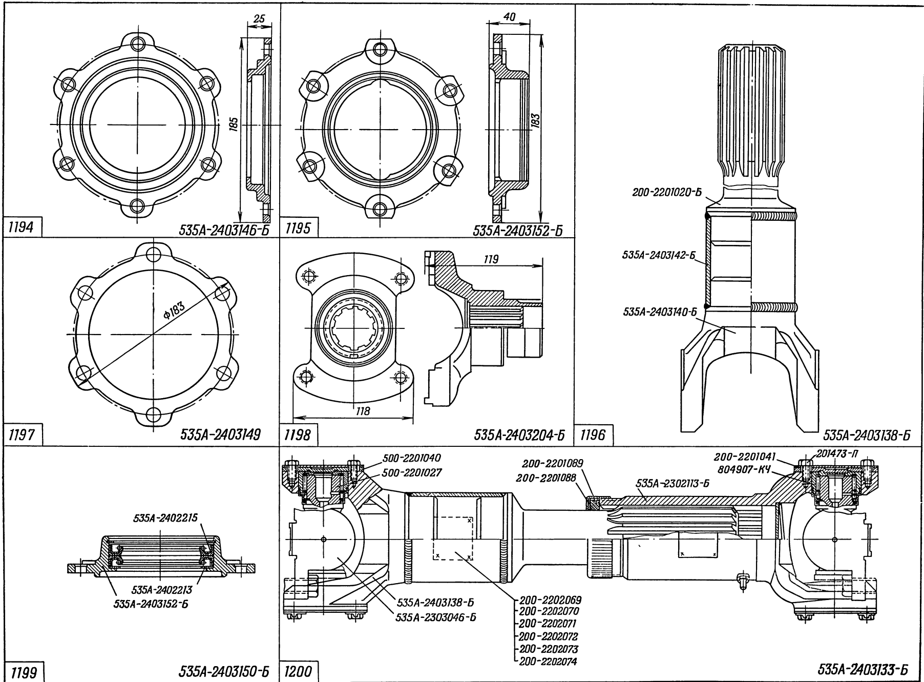
На рис. 1200 вместо дет. 500-2201027 читать дет. 500-2201027-А и вместо дет. 535А-2302113-Б — дет. 535А-2303113-Б
