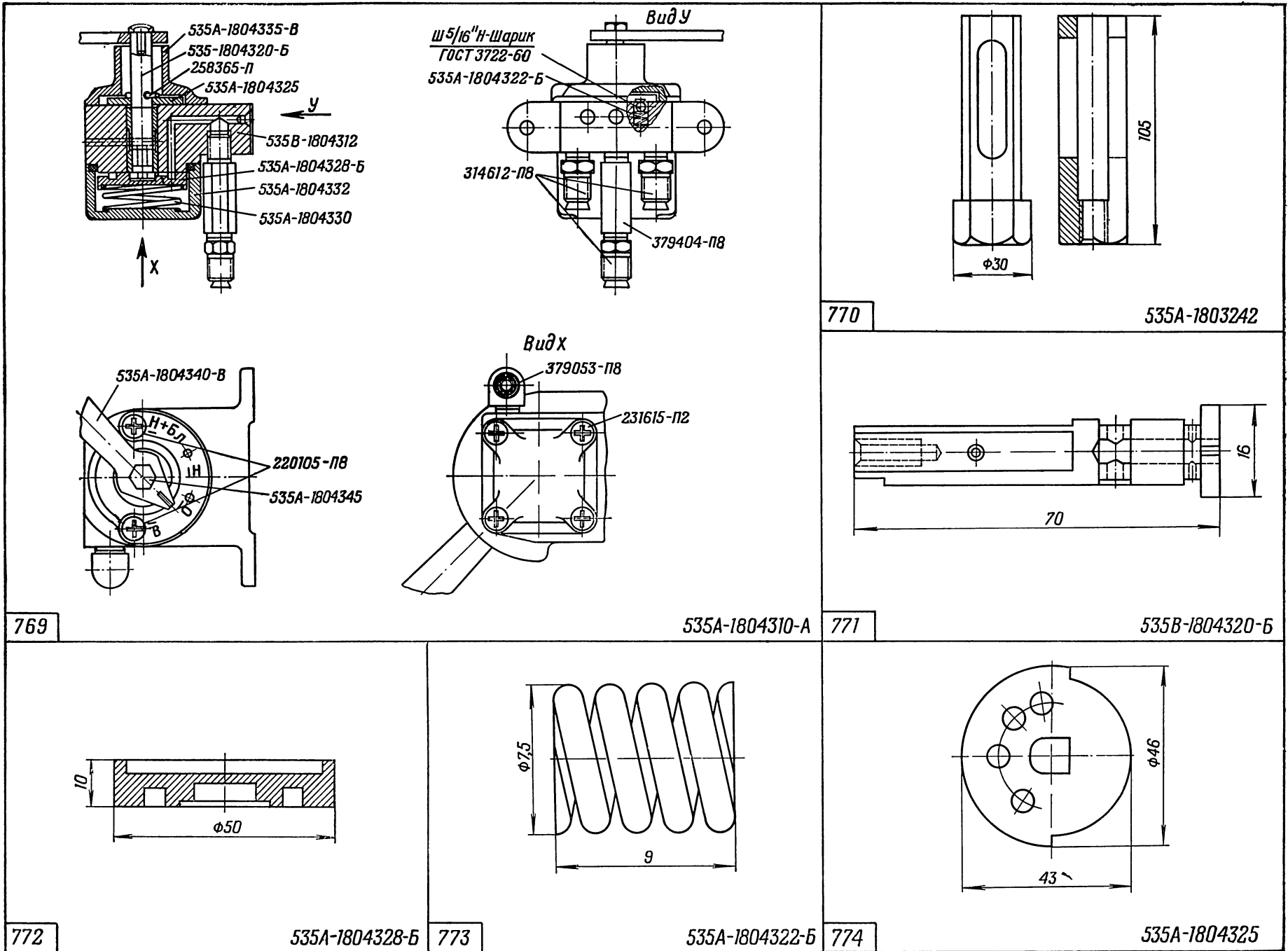
На рис. 769 вместо дет. 535-1804320-Б и на рис. 771 вместо дет. 535B-1804320-Б читать дет. 535A-1804320-Б
