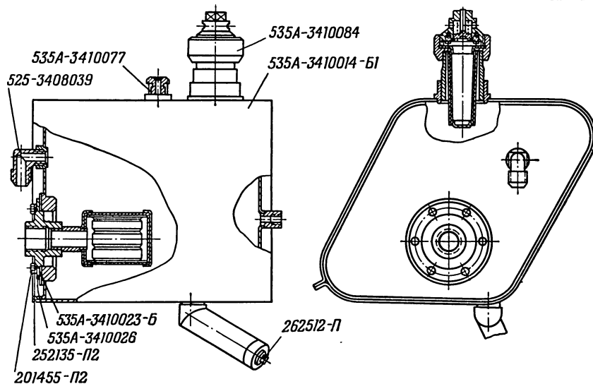
На рис. 1670 изображена дет. 535A-3410014-61
