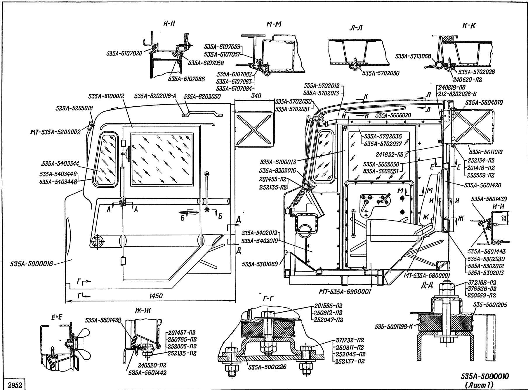
На рис. 2952 вместо дет. 535A-5403344 читать дет. 535A-5403444
