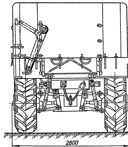
Автомобиль-тягач МАЗ-535А
