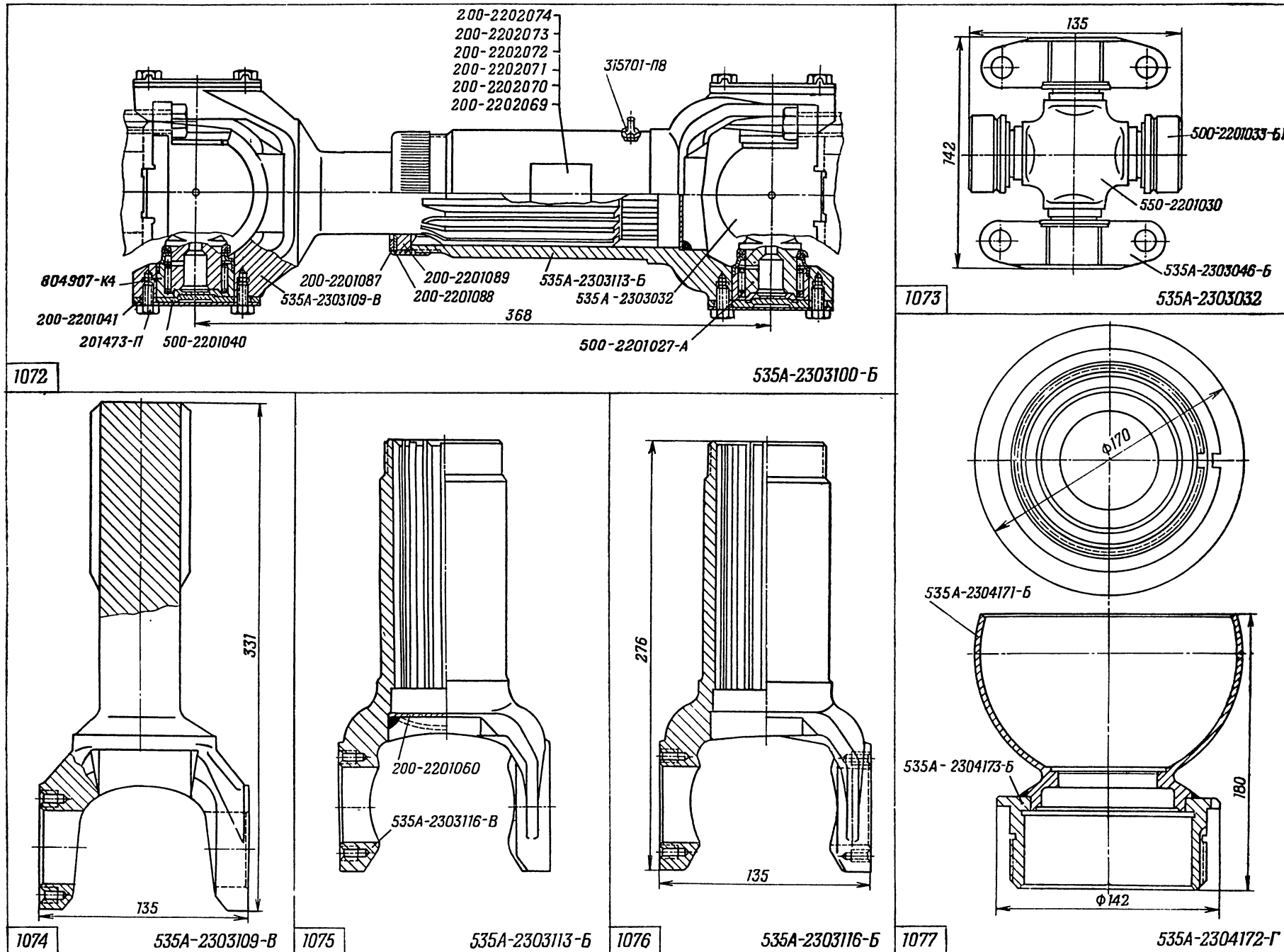
На рис. 1073 вместо дет. 500-2201033-Б1 читать дет. 804907К4 и вместо дет. 550-2201030 — дет. 500-2201030-А
