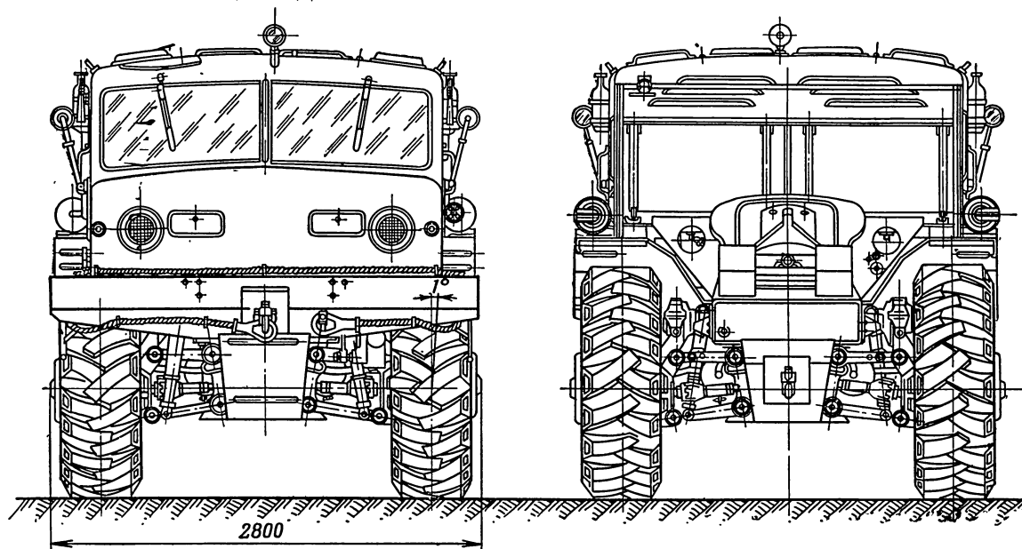
Автомобиль-тягач МАЗ-535В
