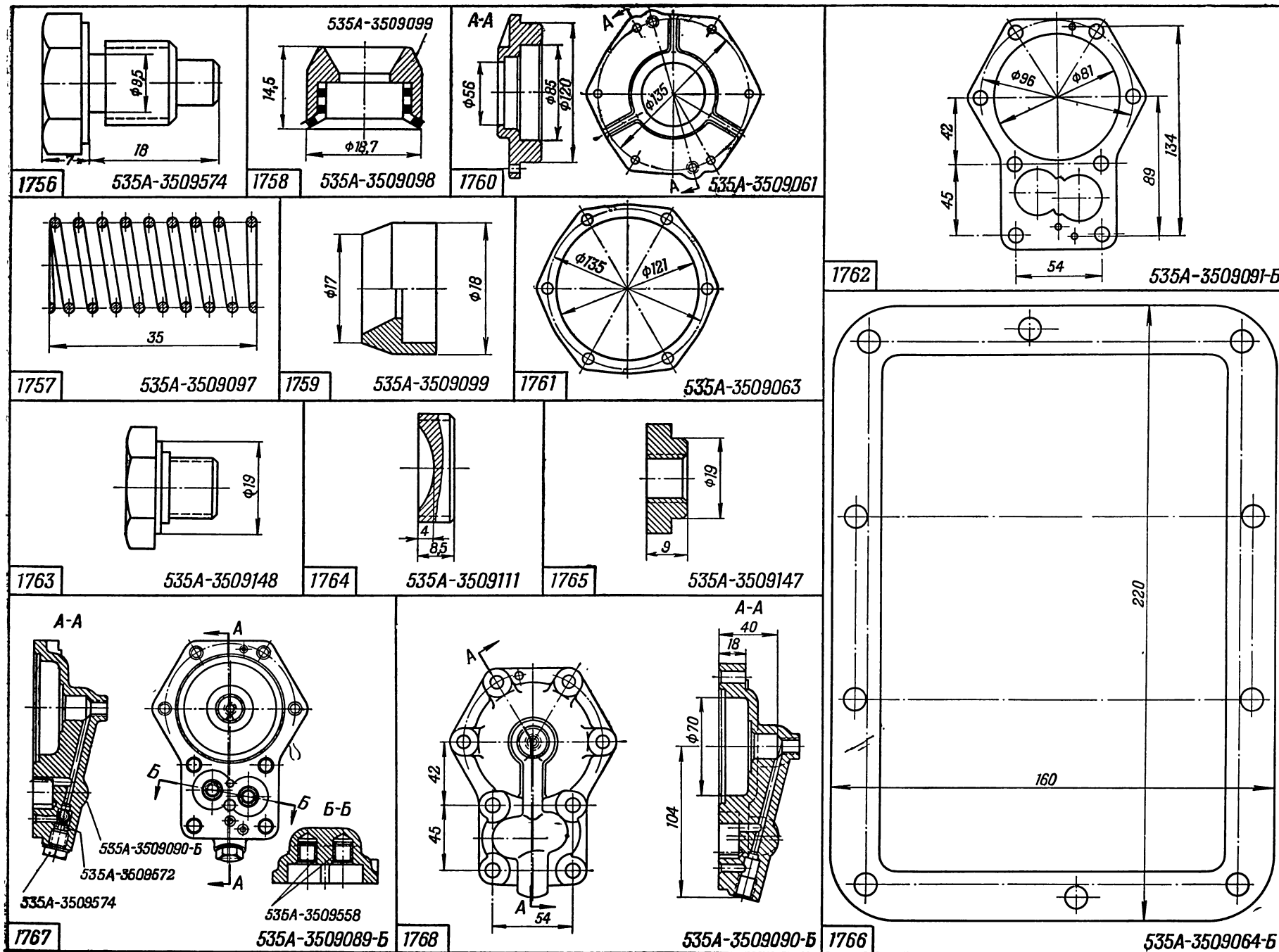
На рис. 1767 вместо дет. 535A-3509558 читать дет. 535A-3509552
