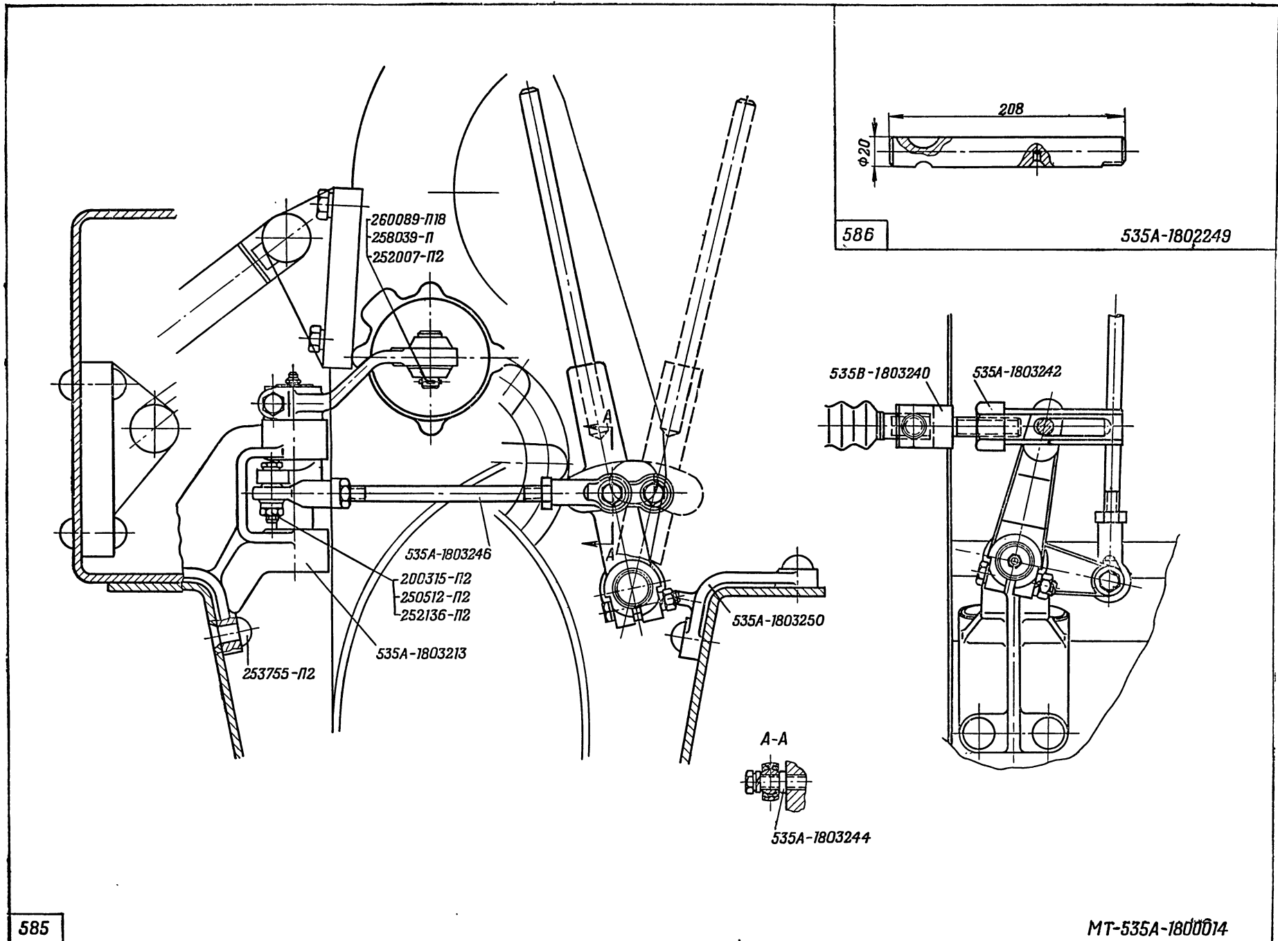
На рис. 585 вместо дет. 535B-1803240 читать дет. 537-1803240
