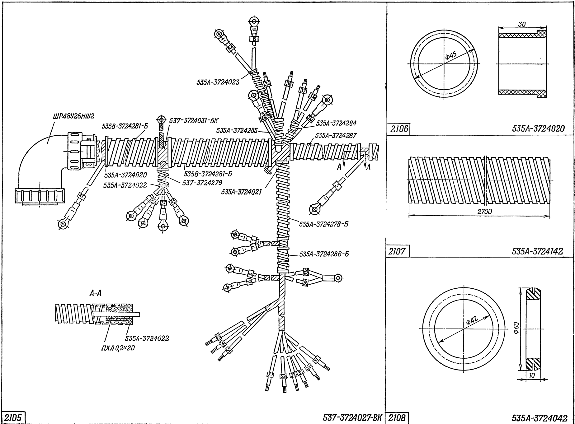
На рис. 2105 вместо дет. 535B-3724281-Б читать дет. 535B-3724282-Б
