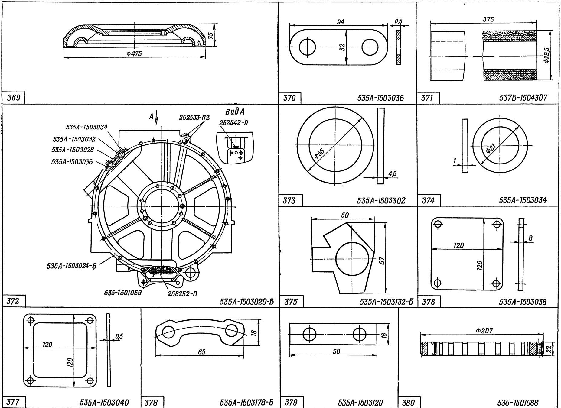
На рис. 369 изображена дет. 535-1501147
