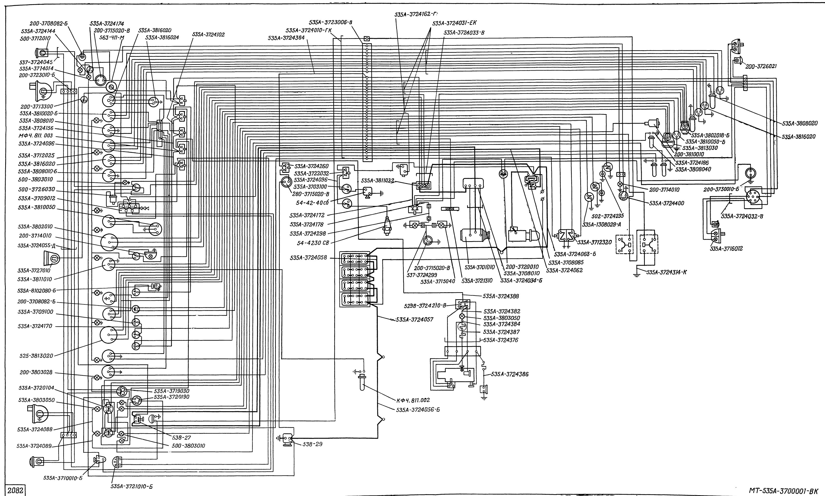
На рис. 2082 вместо дет. 535А-3724058 читать дет. 535А-3724058-А, вместо дет. 535А-3724010-ГК — дет. 535А-3724010-ДК, вместо дет. 535А-3724031-ЕК — дет. 535А-3724031-ЖК и вместо дет. 535А-3724033-В — дет. 535А-3724033-Г
