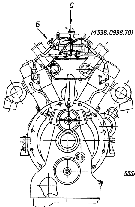
Вид А
