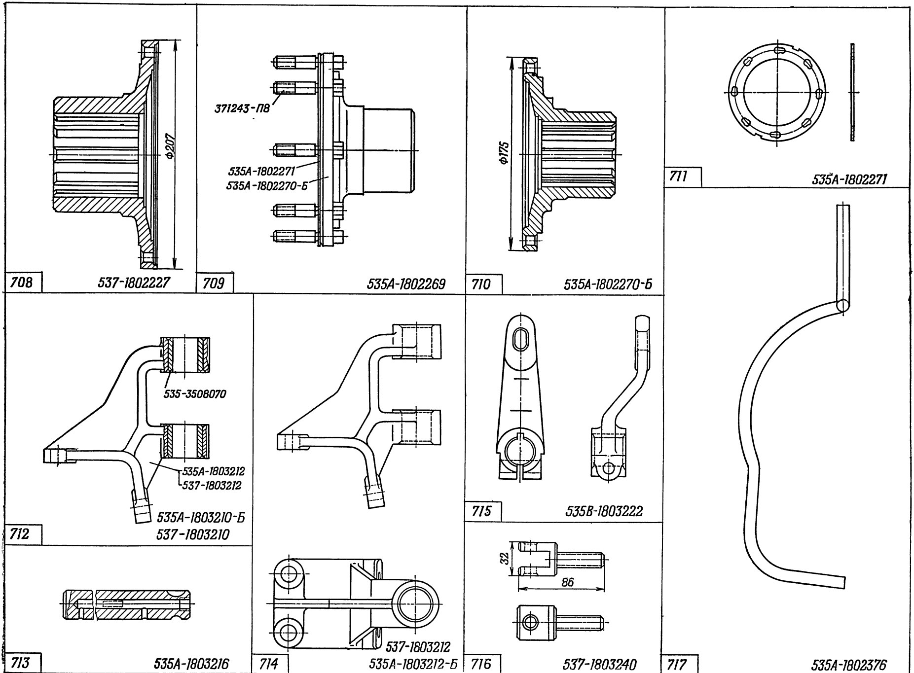
На рис. 712 вместо дет. 535A-1803212 читать дет. 535A-1803212-Б
