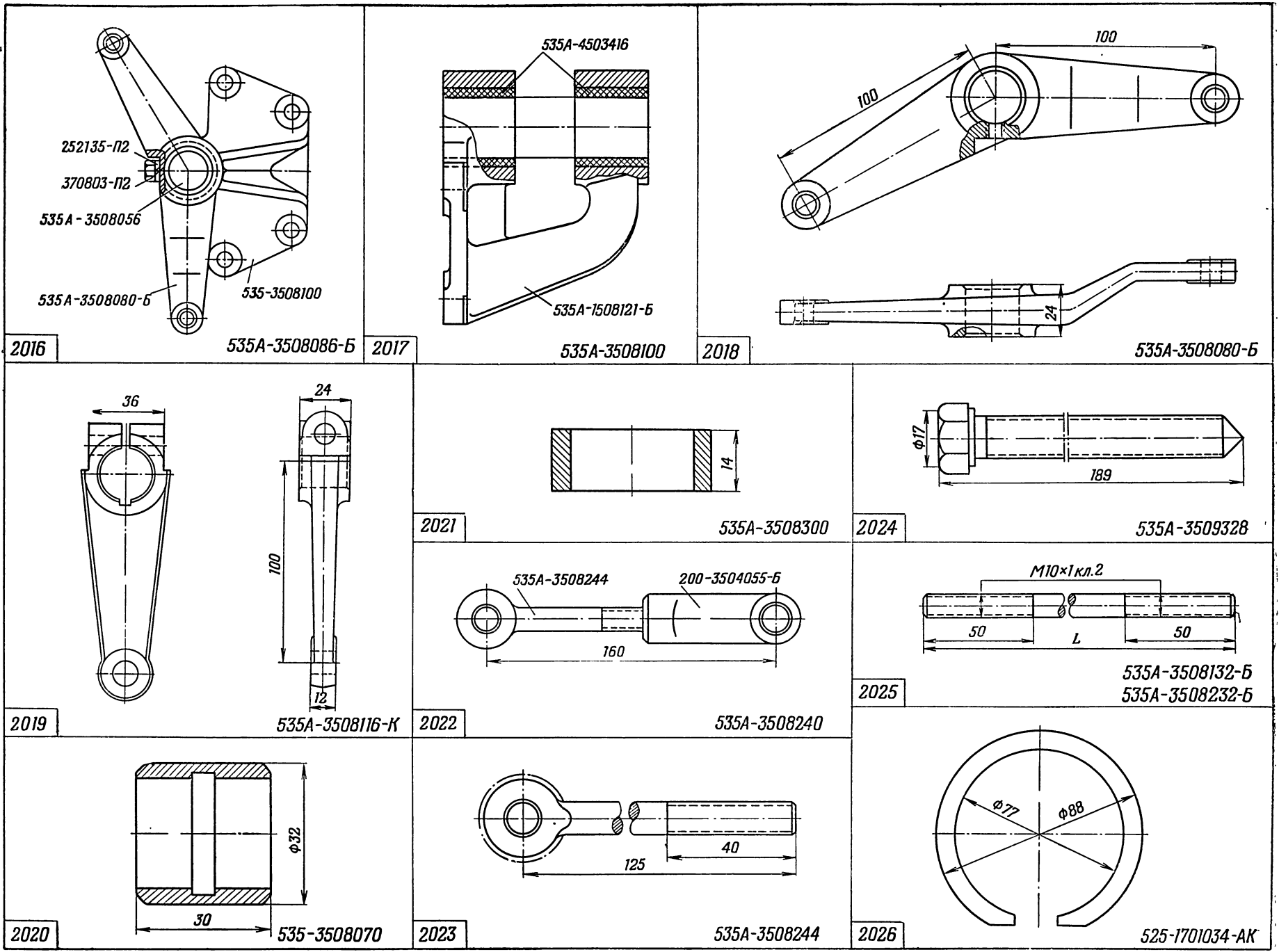
На рис. 2016 вместо дет. 535-3508100 читать дет. 535A-3508100
