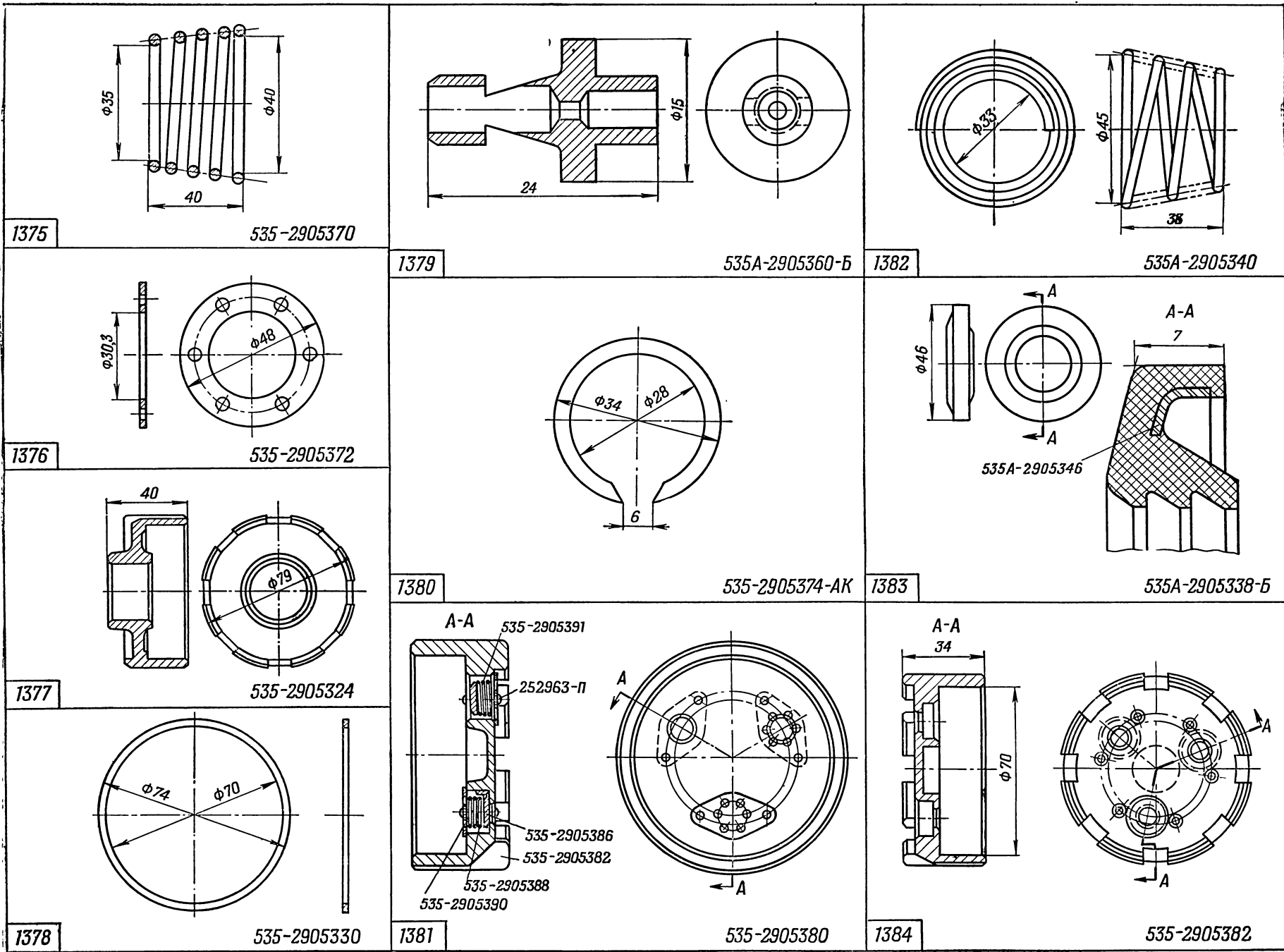
На рис. 1381 вместо дет. 535-2905391 читать дет. 535-2905394
