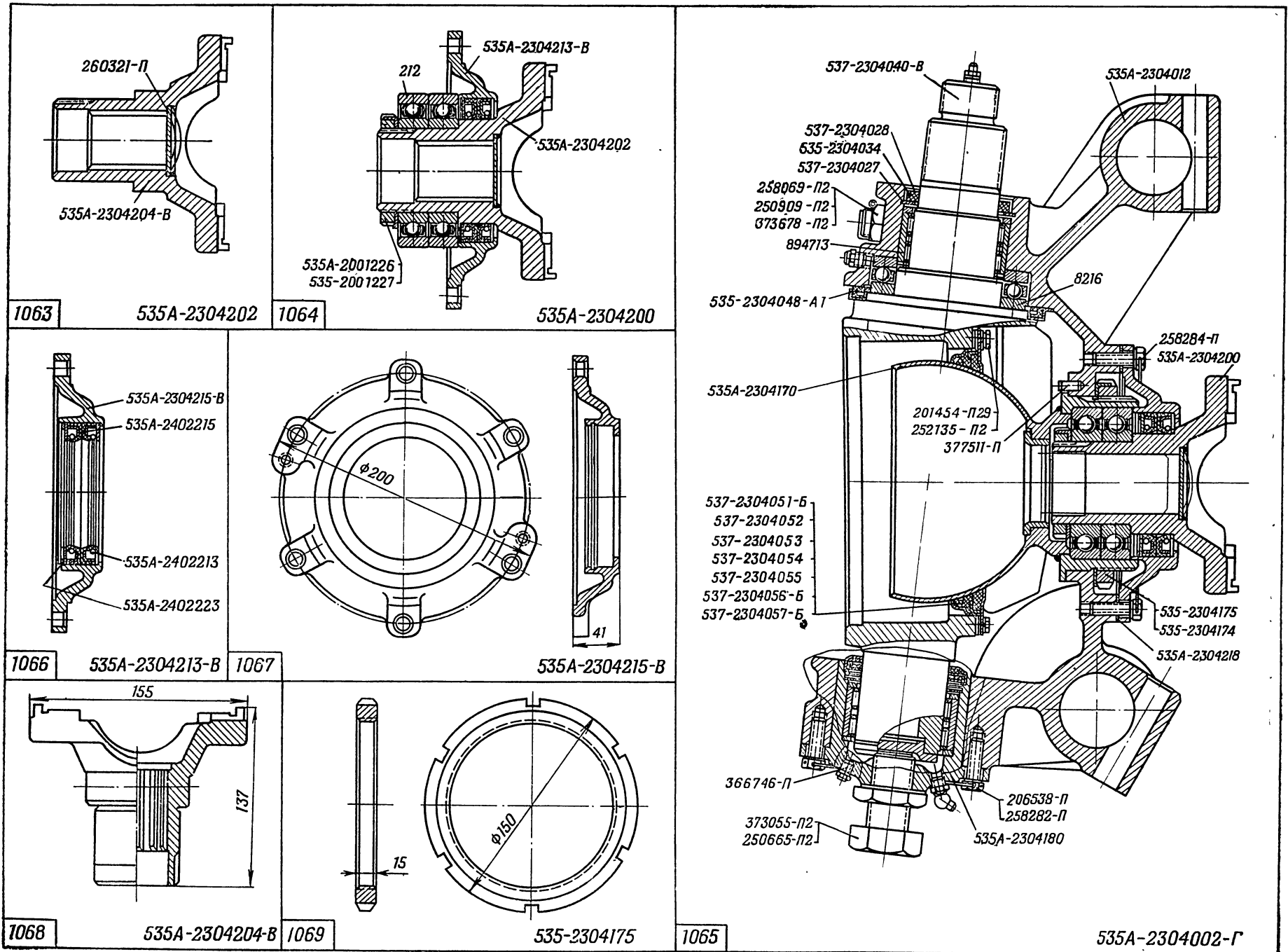
На рис. 1065 вместо дет. 537-2304052 читать дет. 537-2304052-А
