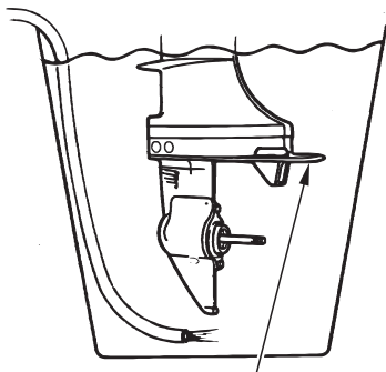
АНТИКАВИТАЦИОННАЯ ПЛИТА
