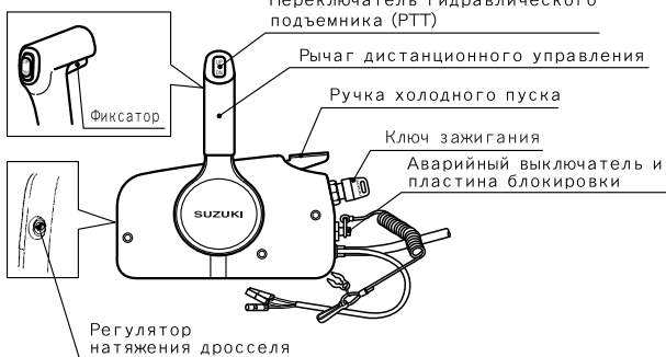
ДИСТАНЦИОННОЕ УПРАВЛЕНИЕ
