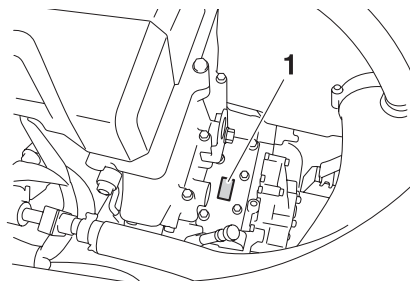
1 Место расположения серийного номера двигателя
