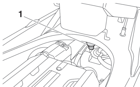
1 Водоотделитель
