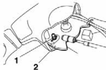
1 Шарнирный болт троса рулевого управления 2 Рулевая колонка
