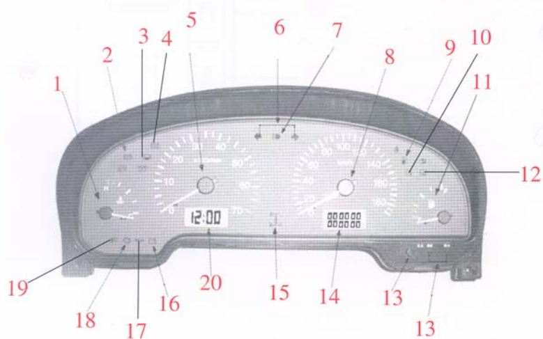
Контрольно-измерительные приборы, сигнализаторы и указатели
