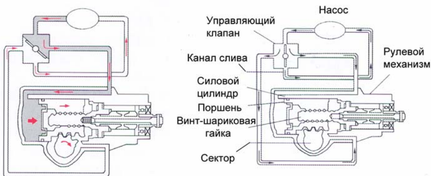
Рис. 12. А. Среднее положение (колеса прямо)
