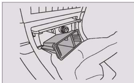
Демонтаж пепельницы.
