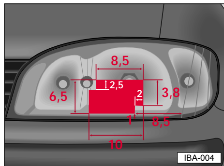
Переход от езды слева на езду справа - левая фара.
