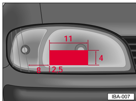
Переход от езды слева на езду справа - правая фара.
