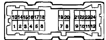
Разъем I
