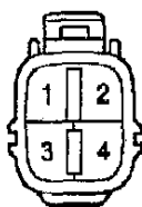
Разъем В
