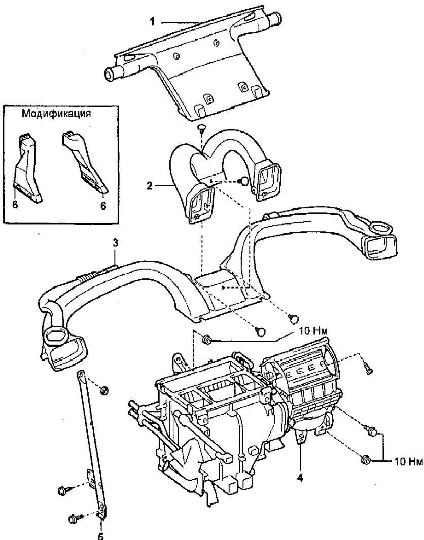
Снятие и установка блока кондиционера и отопителя. 1 - дефлектор обдува лобового стекла, 2 - воздуховод №2, 3 - воздуховод №1, 4 - блок кондиционера и отопителя, 5 - стойка усилителя панели приборов, 6 - воздуховод №3.
