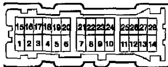
Разъем H
