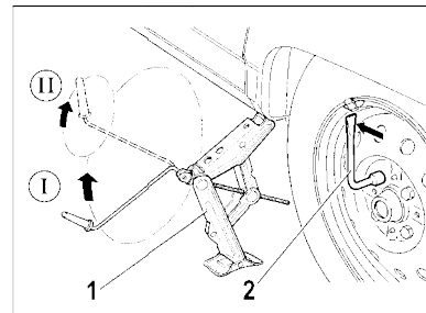
Рис. 42. Подъем автомобиля при замене колес
