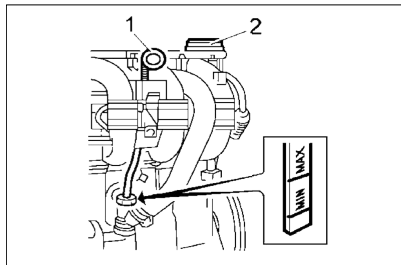
Рис. 33. Проверка уровня масла в картере двигателя
