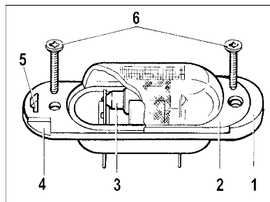
Рис. 49. Фонарь освещения номерного знака
