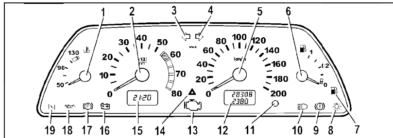
Рис. 21. Комбинация приборов
