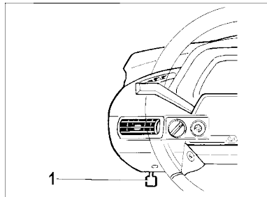
Рис. 14. Рукоятка привода замка капота
