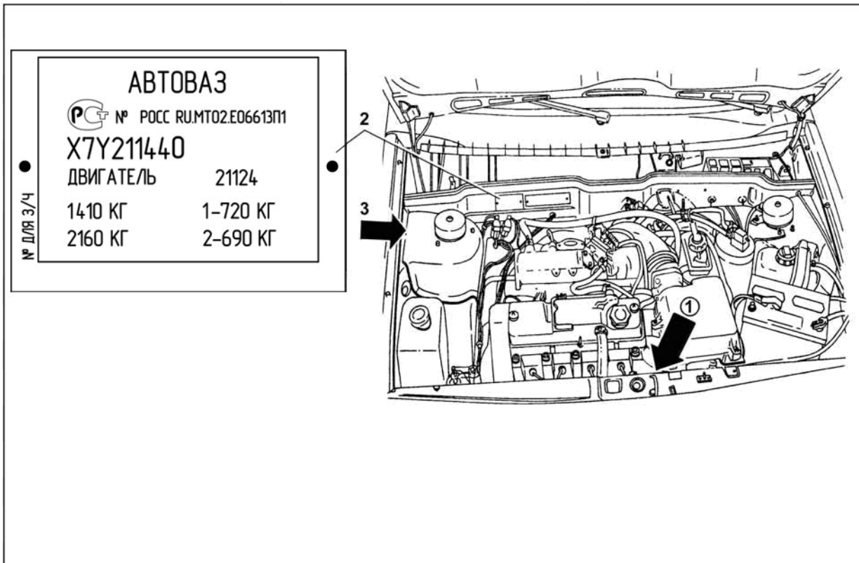
Рис. 55. Паспортные данные
