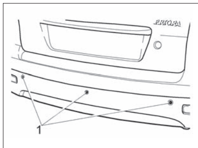
Рис. 73. Датчики парковки
