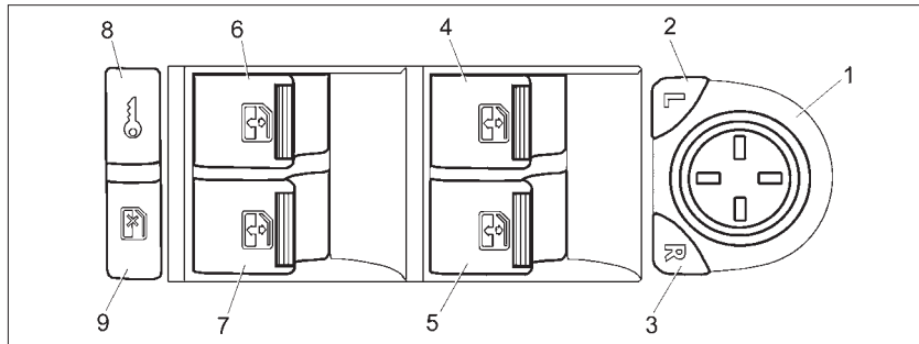
Рис. 10. Модуль двери водителя
