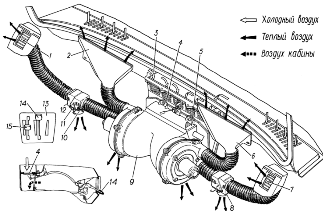
Рис. 8.1. Отопитель кабины:
