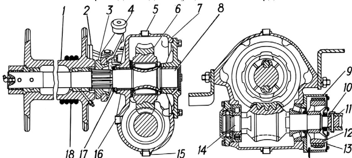
Рис. 8.5. Лебёдка с редуктором:
