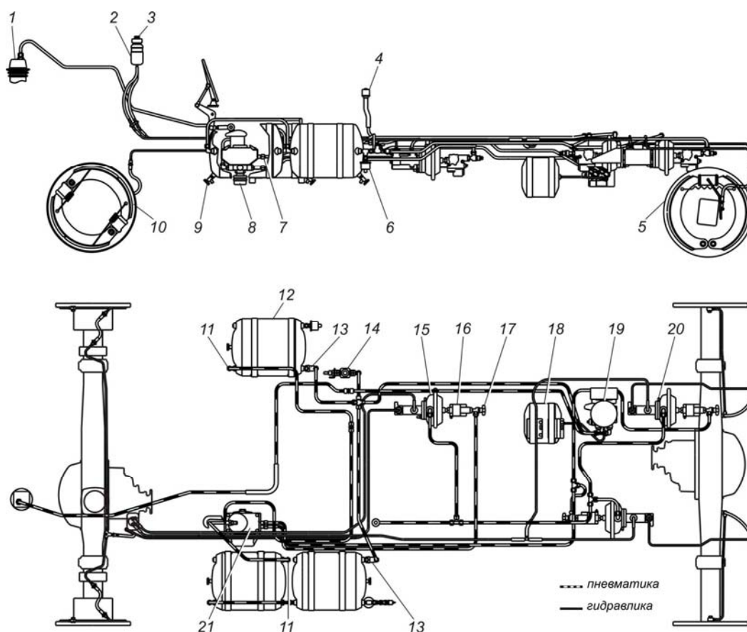
Рис. 8.3. Принципиальная схема рабочей тормозной системы автомобилей с ABS:
