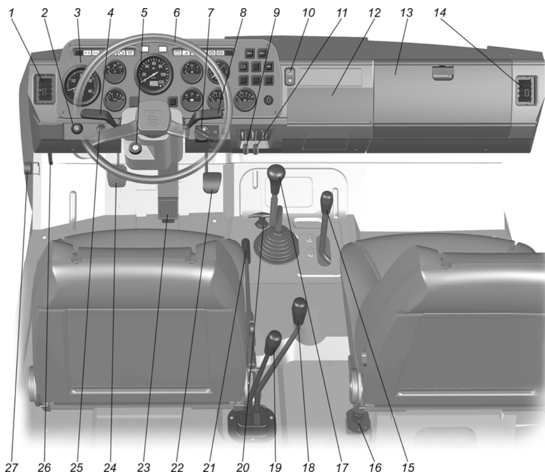
Рис. 5.1. Органы управления
