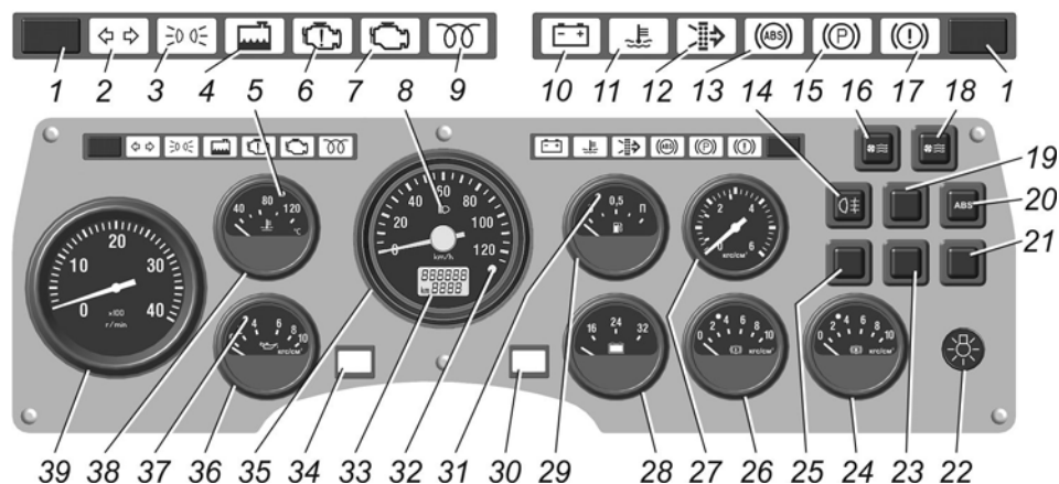
Рис. 5.13. Щиток приборов автомобиля ГАЗ-33088:
