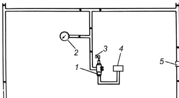
Рис. 8.4. Схема системы регулирования давления в шинах:
