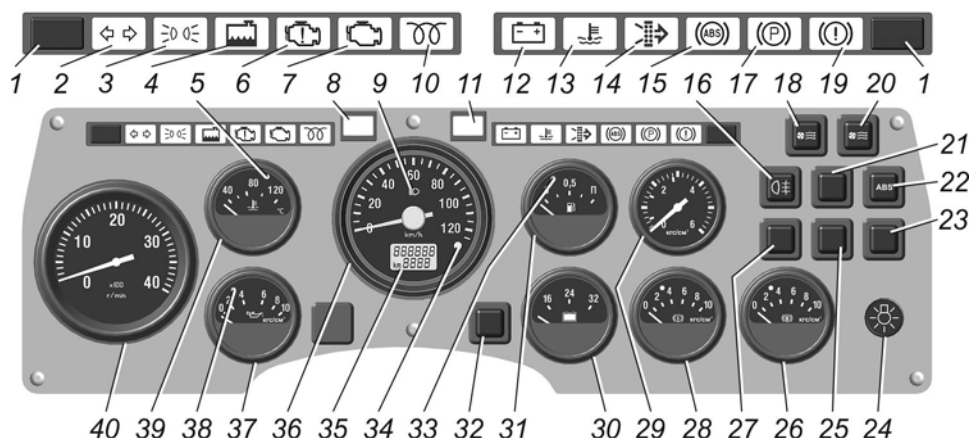
Рис. 5.12. Щиток приборов автомобиля ГАЗ-33081 с двигателем ММЗ Д-245.7 ЕЗ:
