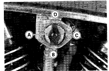
A. Fuel Tap B. ON position C. PRI position D. RES position
