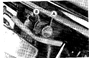
A. Choke Knob B. Locknut
