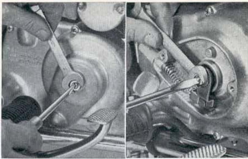
Koppeling-steischroef en borgmoer (model C 100 en C 102).
