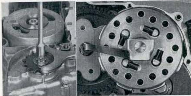
Afnemen van het lettingtandwiel Koppeling, oliebakje (model C 110 en C 114). (alle modellen).
