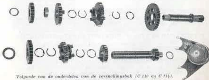
Volgorde van de onderdelen van de versnellingsbak (C 110 en C 114).
