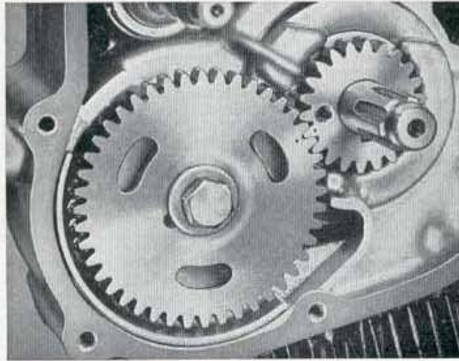
Distributieafstelling (kleppen) (alle modellen).
