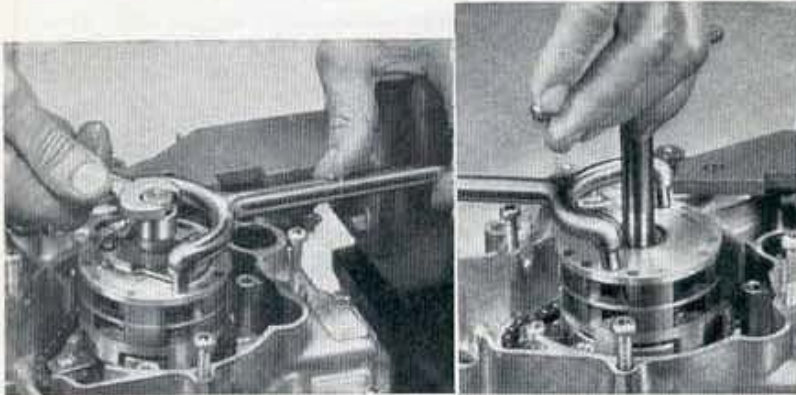
Vasthouden van de rotor met het speciale gereedschap om de bout te kunnen losdraaien.
