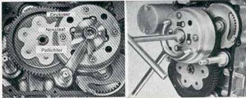
Koppelingsmechanisme, aandrijftandwiel, olieplaat en nokkenas.
