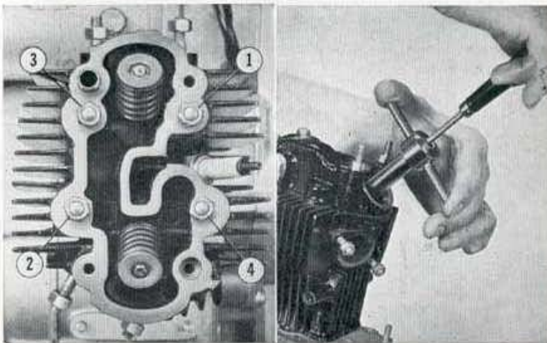
Volgorde voor het vastzetten van de cilinderkop.
