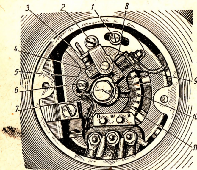
Фиг. 34. Прерыватель:
