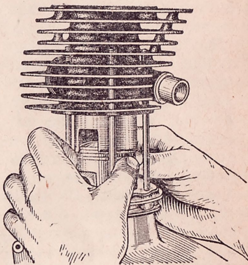
Фиг. 16. Монтаж цилиндра.
