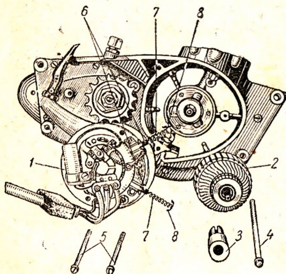
Фиг. 33. Генератор в разобранном виде:
