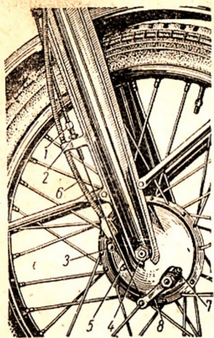
Фиг. 26. Привод тормоза переднего колеса:
