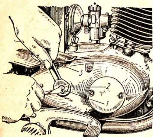
Фиг. 18. Регулировка сцепления:
