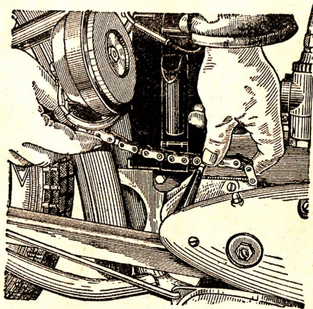
Фиг. 24. Надевание цепи на ведущую звездочку.
