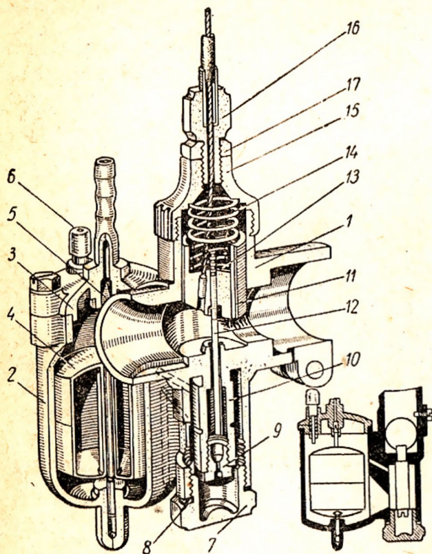
Фиг. 12. Карбюратор:
