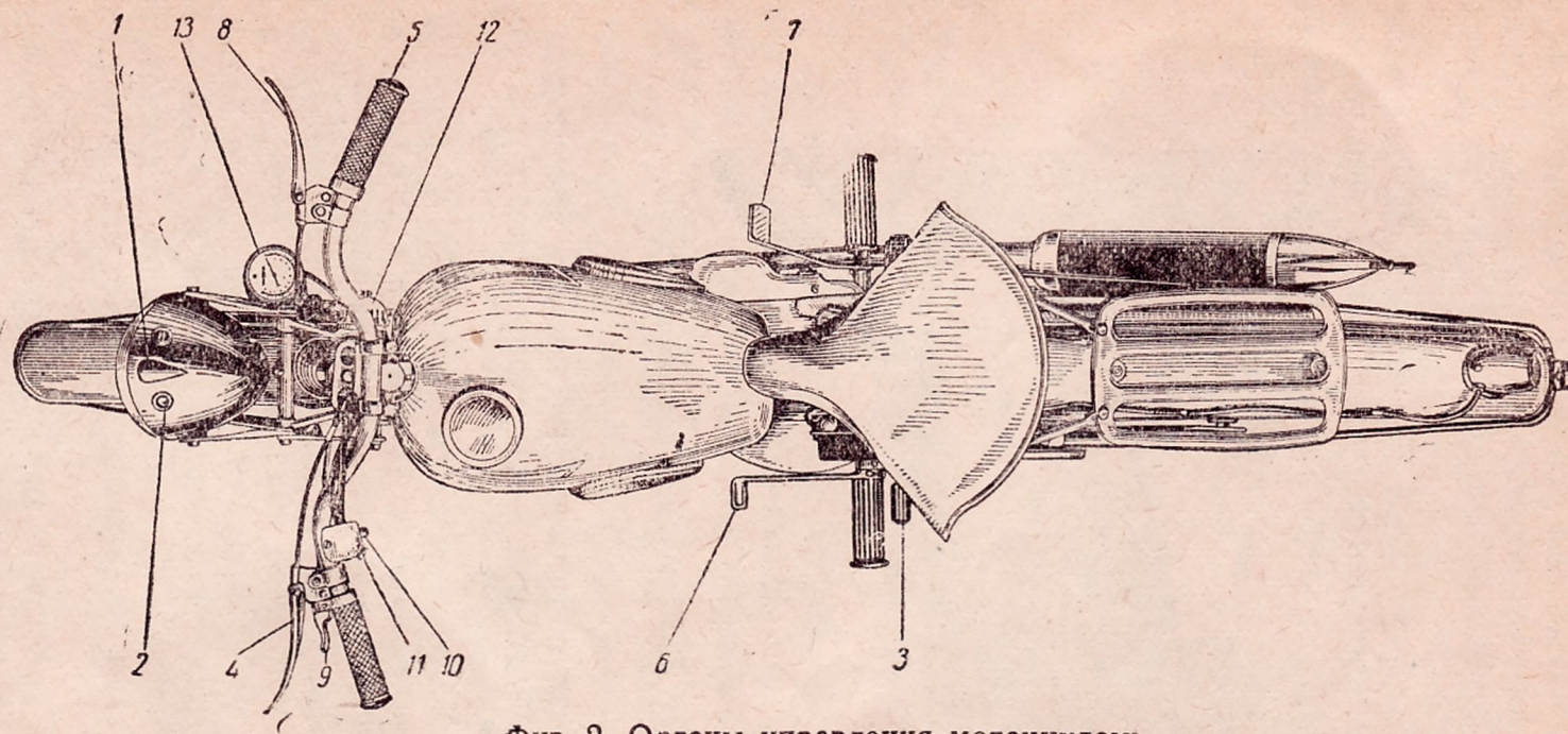
Фиг. 2. Органы управления мотоциклом:
