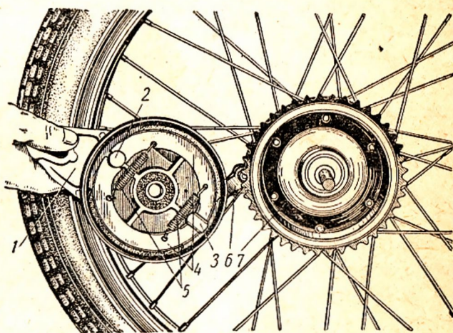
Фиг. 27. Тормоз заднего колеса:
