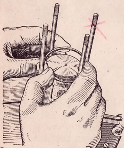
Фиг. 15. Снятие поршневых колец.
