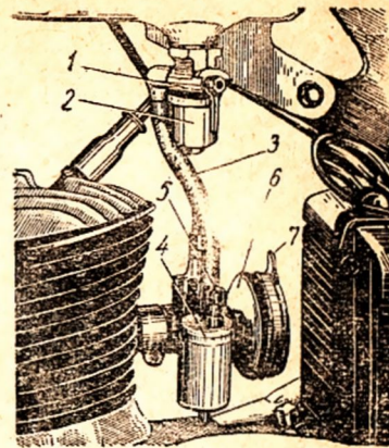
Фиг. 10. Система питания:
