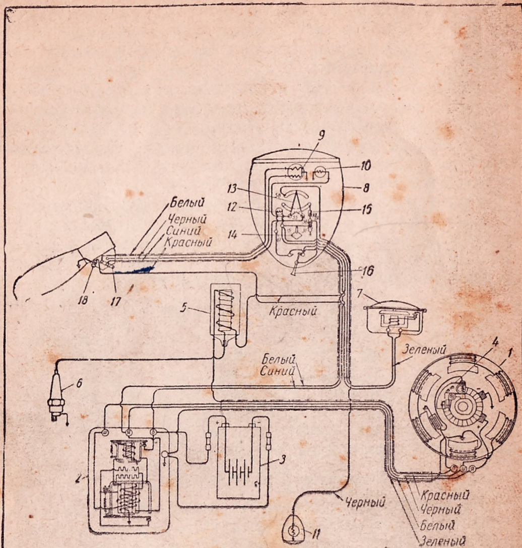
Фиг. 31. Схема электрооборудования:
