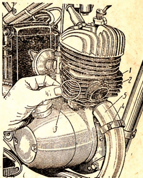
Фиг. 13. Крепление выпускной трубы к цилиндру:
