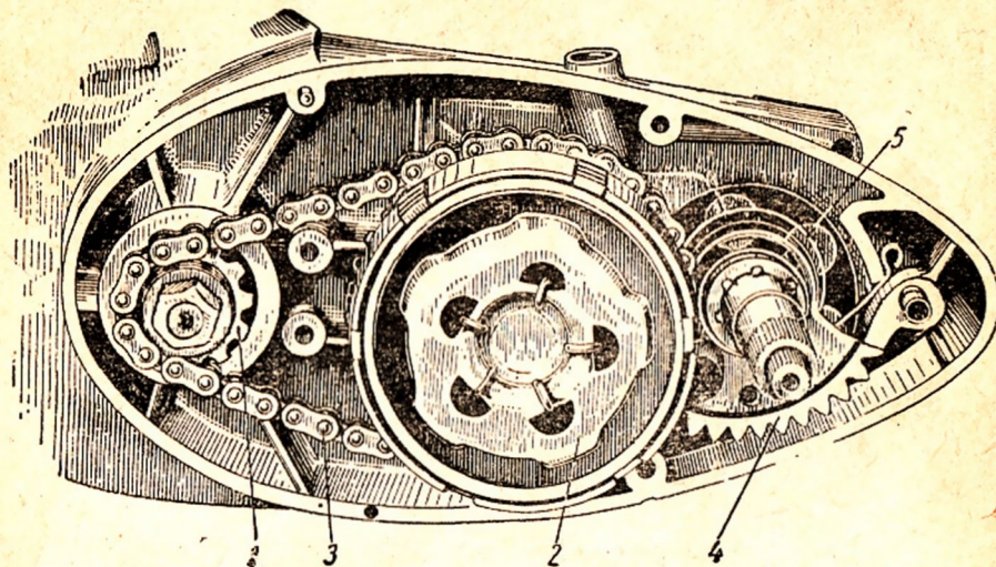
Фиг. 17. Привод коробки передач:
