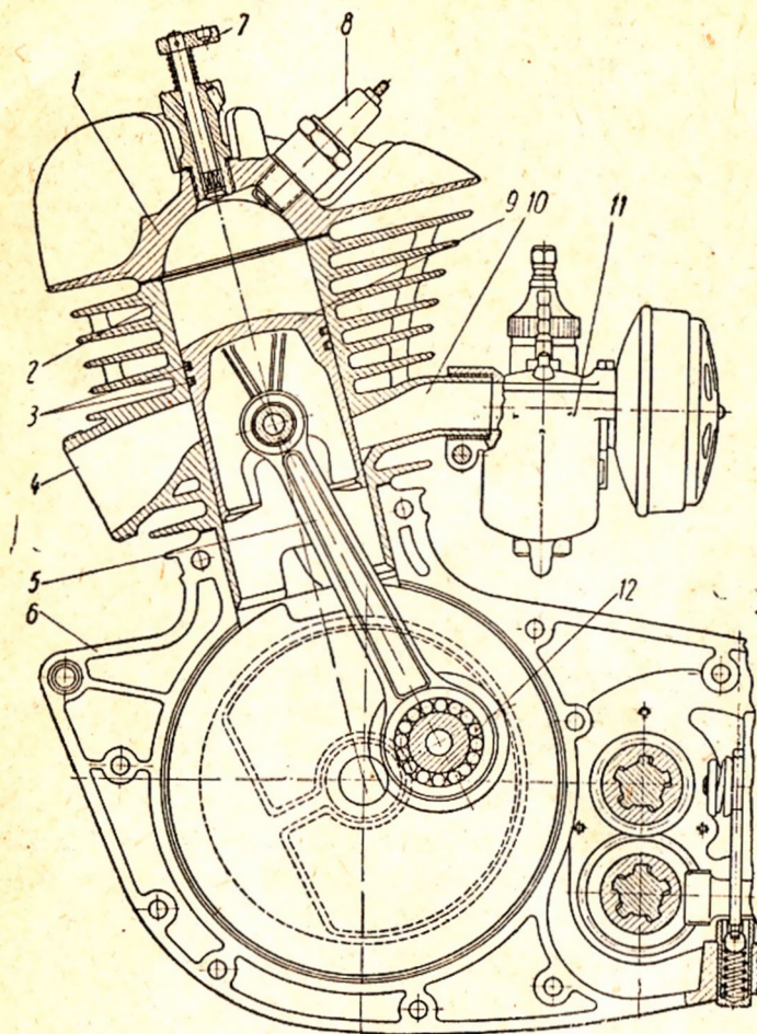
Фиг. 7. Продольный разрез двигателя:
