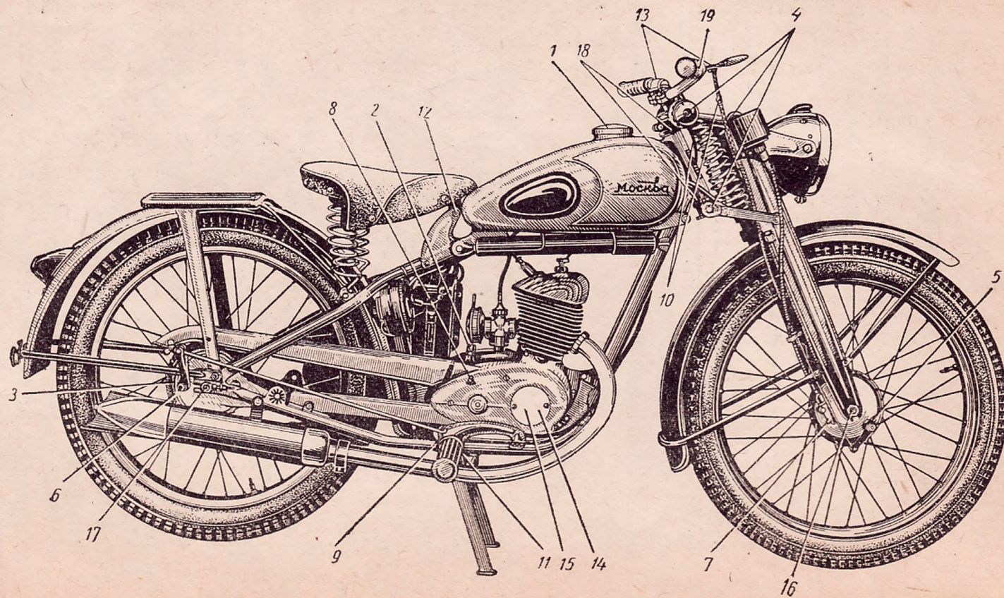
Фиг. 36. Схема смазки.
