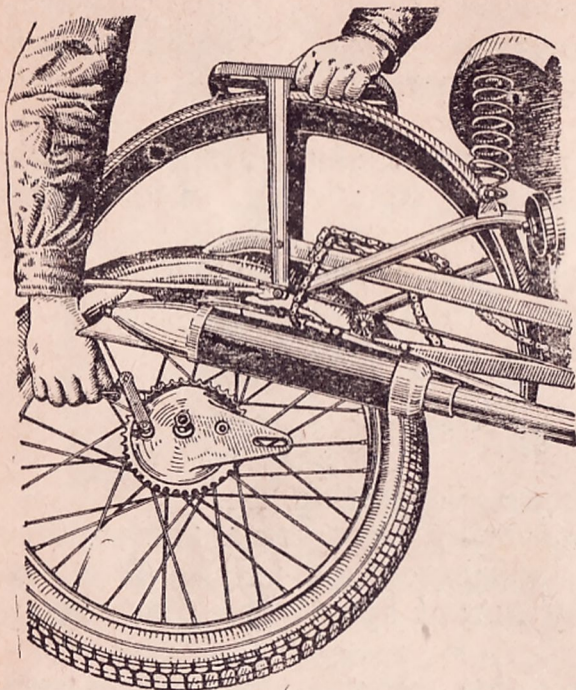
Фиг. 28. Снятие заднего колеса.
