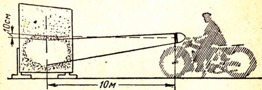
Фиг. 35. Схема установки фары.
