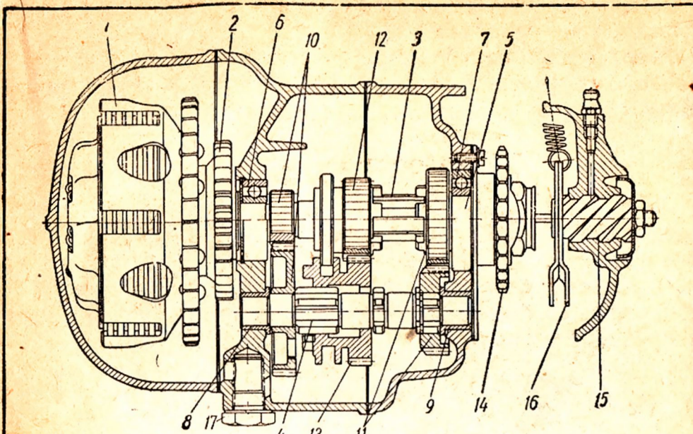
Фиг. 19. Коробка передач:
