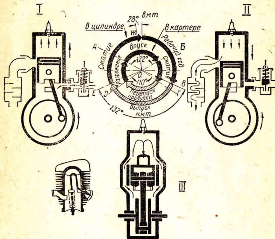
Фиг. 9. Рабочий процесс двигателя:
