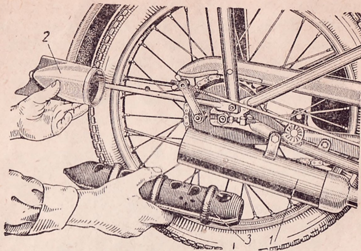
Фиг. 14. Глушитель:
