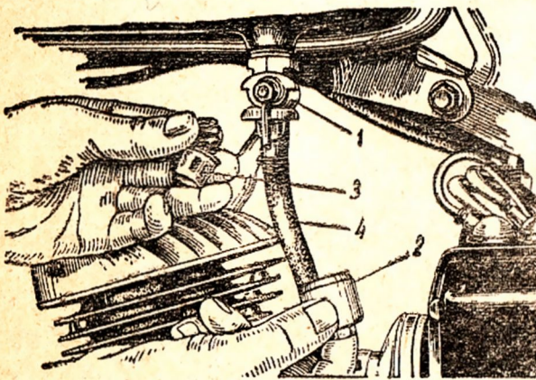
Фиг. 11. Чистка топливного фильтра:
