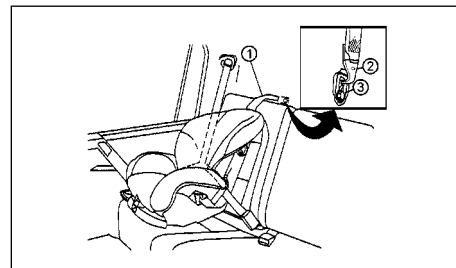
Заднее сиденье-диван
