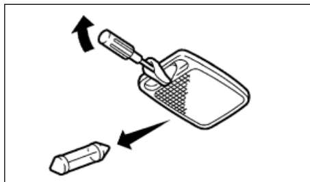
Плафон освещения задней части кабины (для некоторых вариантов исполнения автомобиля)
