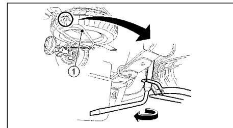
Кронштейн крепления запасного колеса (для некоторых вариантов исполнения автомобиля)
