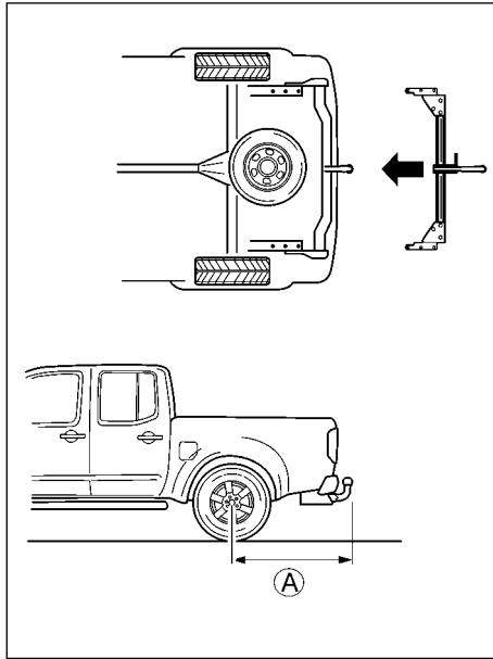
Автомобили с кабиной Double Cab
