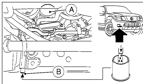
Масляный фильтр - двигатель V9X
