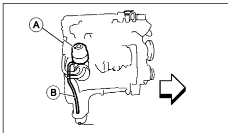
Масляный фильтр - двигатель YD
