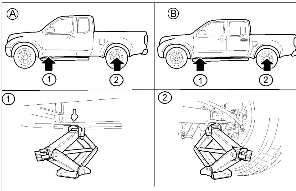
Места расположения опор домкрата
