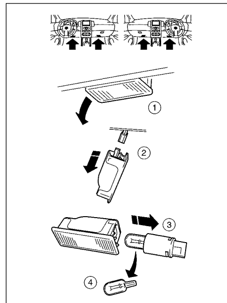
Плафоны подсветки пола кабины (для некоторых вариантов исполнения автомобиля)
