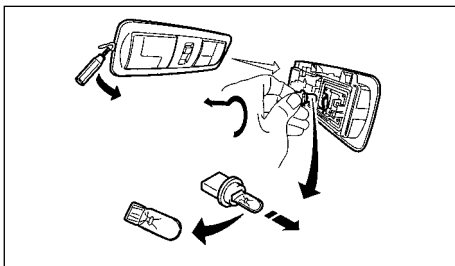
Плафоны общего и местного освещения (тип А, для некоторых вариантов исполнения автомобиля)
