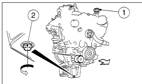
Сливная пробка - двигатель V9X
