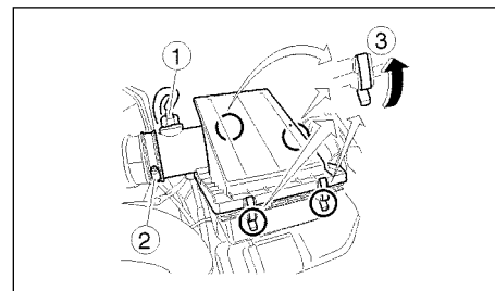
Двигатель YD или V9X
