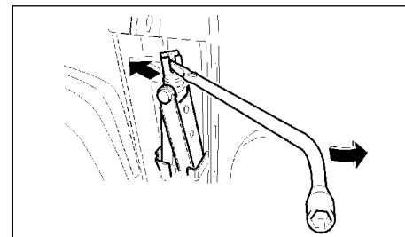
Автомобили с кабиной "King Cab"
