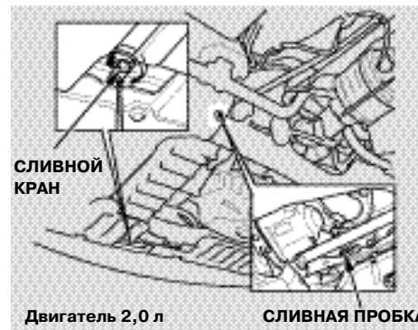
СЛИВНАЯ ПРОБКА
