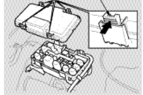
ПОДКАПОТНАЯ КОРОБКА ЛАПКА ФИКСАТОРА ПРЕДОХРАНИТЕЛЕЙ
